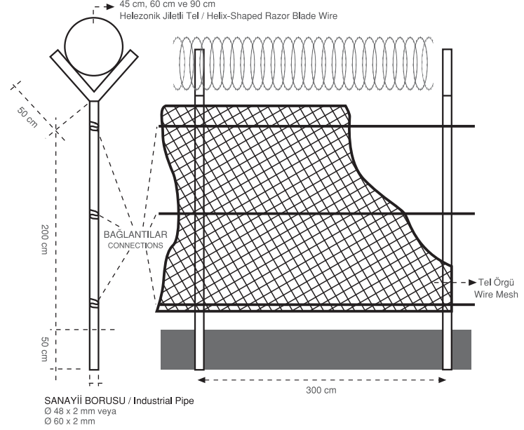
Boru Direkli Tel Çit Üzeri Helezonik Jiletli Tel Uygulaması Spiral Razor Wire Application over Wire Fence With Pipe Pole
