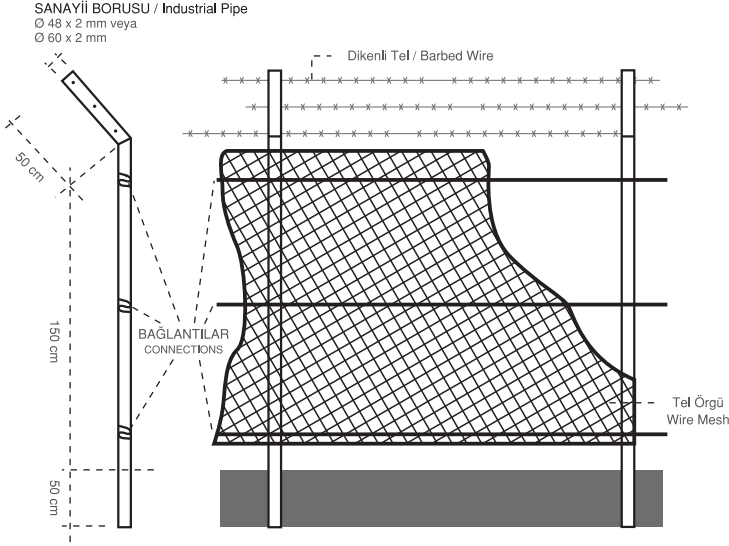
Boru Direkli Tel Çit Üzeri Dikenli Tel Uygulaması (200 cm) Barbed Wire Application over Wire Fence With Pipe Pole (200 cm)
