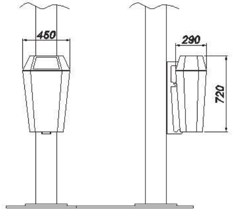
Prizmatik Tip Çöp Kovası Prismatic Type Litter Bin
