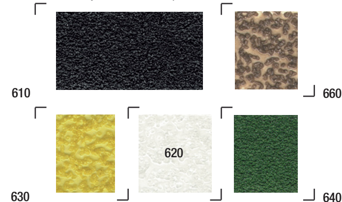
3M™ Safety-Walk™ prilagodljiva na oblik
