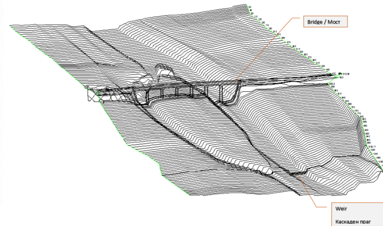
3D multiple cross section plot / 3D приказ на попречните профили
