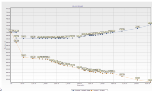
ХИДРАУЛИЧКИ НАДОЛЖЕН ПРОФИЛ НА ХДЛ ВО НИСКА ЗОНА ОД КАПТАЖИ ДО ПУМПНИ СТАНИЦИ ПРИ МАКСИМАЛНА ЧАСОВА ПОТРОШУВАЧКА (12 ЧАСОТ)
