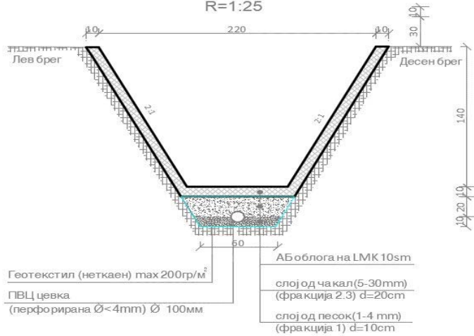
Типски дренажен трапезен канал R=1:25
