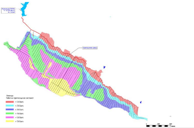
Слика 8.1: Работни притисоци во мрежата а наводнување при гравитационен довод
