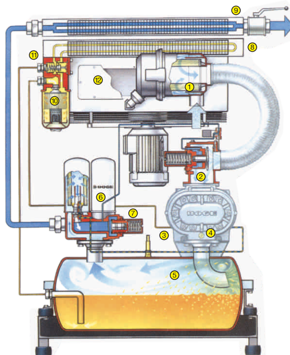
Принцип на работа на завојните компресори
